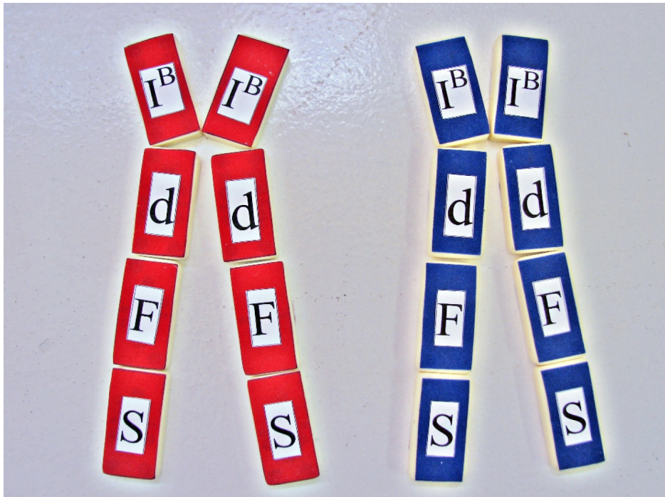
Figura 2: Representação de um par de cromossomos homólogos com quatro loci, organizados de maneira linear, referente à sugestão utilizada de atividade com o indivíduo 1.
