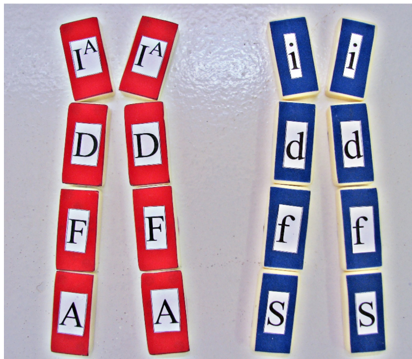
Figura 5: Representação de um par de cromossomos homólogos, com todos os loci em heterozigose, referente à sugestão utilizada de atividade com o indivíduo 2.
